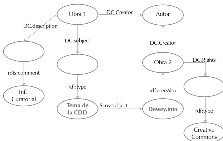
Figura 3. Ejemplo de organización de colecciones basada en la Clasificación Decimal Dewey y datos enlazados por estructuras Resource Description Framework
